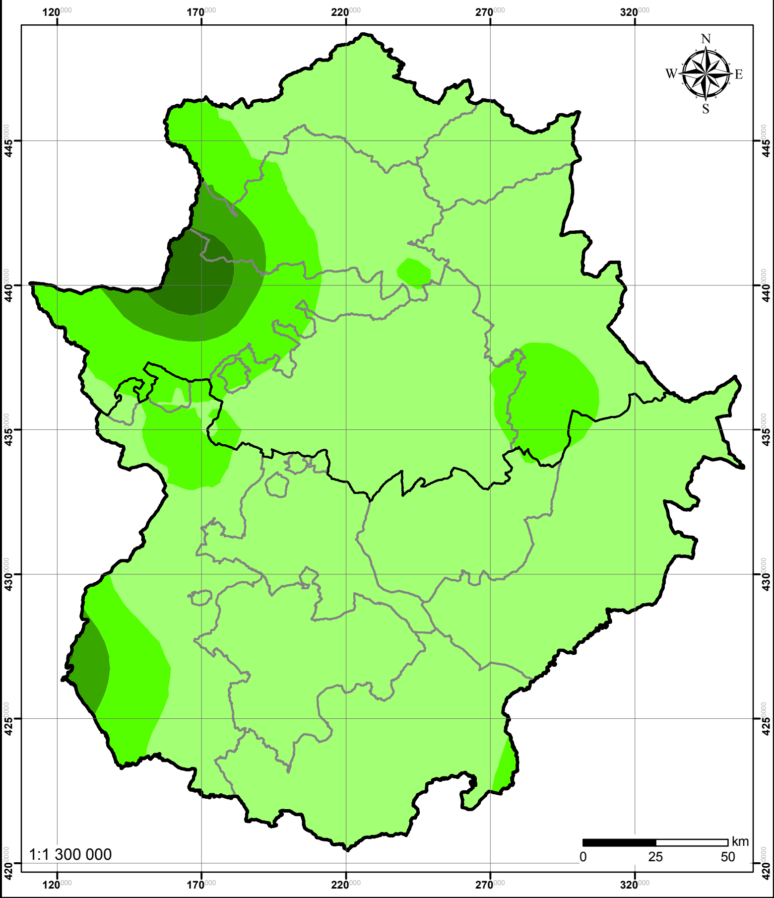
Mapa 29. Variación de la temperatura media anual de las mínimas diarias en el año 2050 respecto del año 2025 (Escenario B2).
