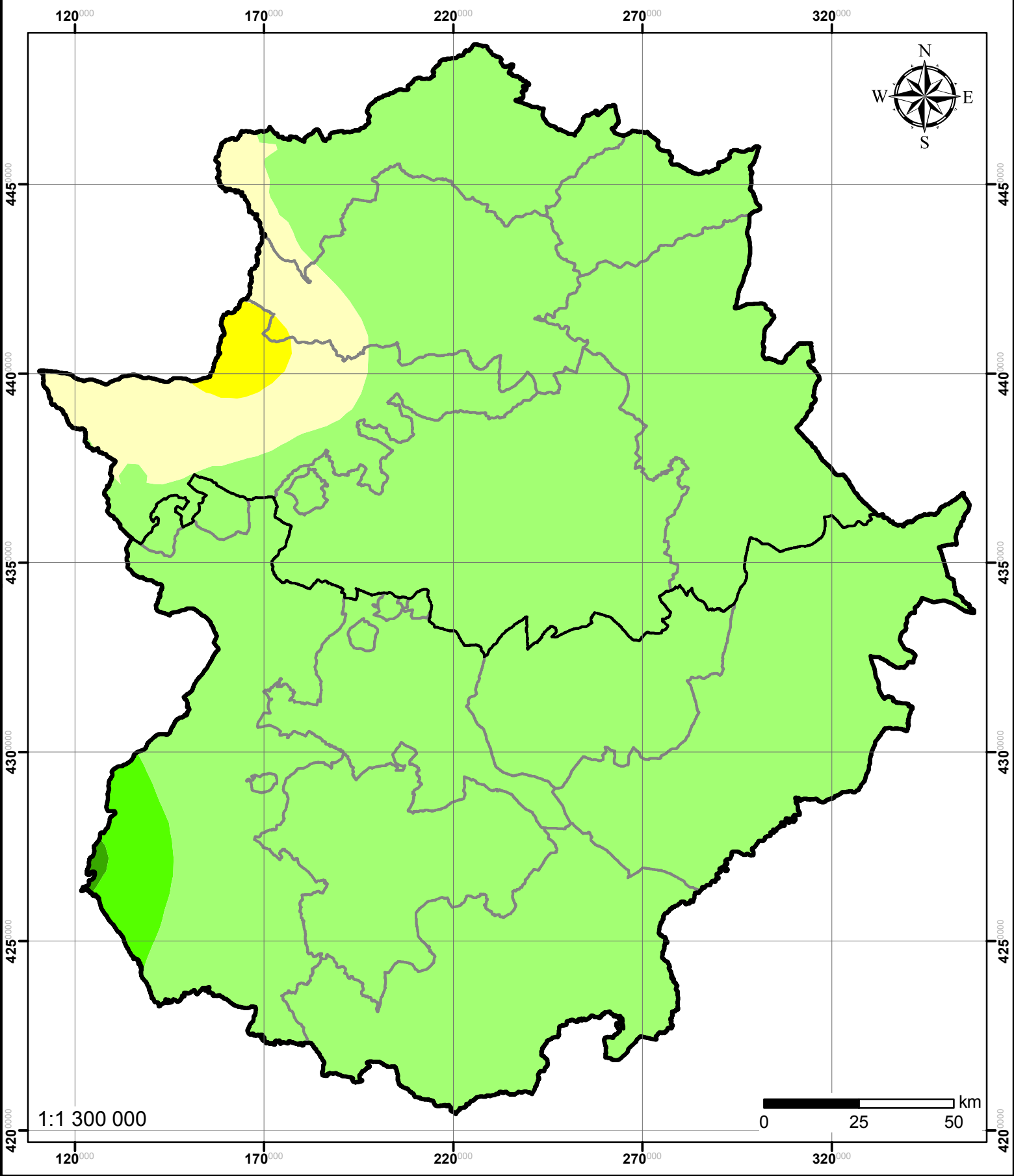
Mapa 28. Variación de la temperatura media anual de las mínimas diarias en el año 2050 respecto del año 2025 (Escenario A2).
