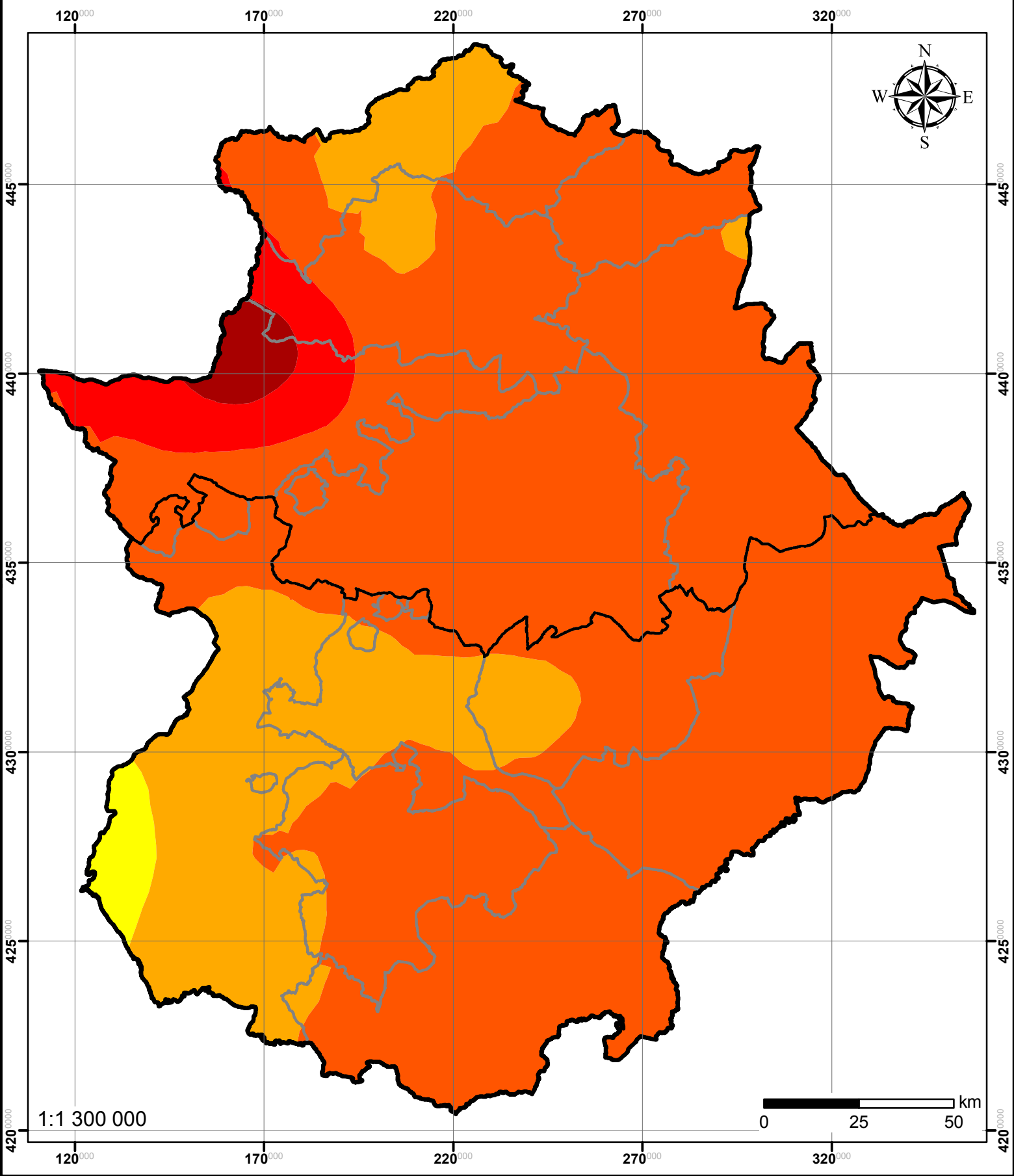
Mapa 26. Aumento de la temperatura media anual de las mínimas diarias en el año 2050 (Escenario A2) respecto del promedio del periodo 1961-1990.
