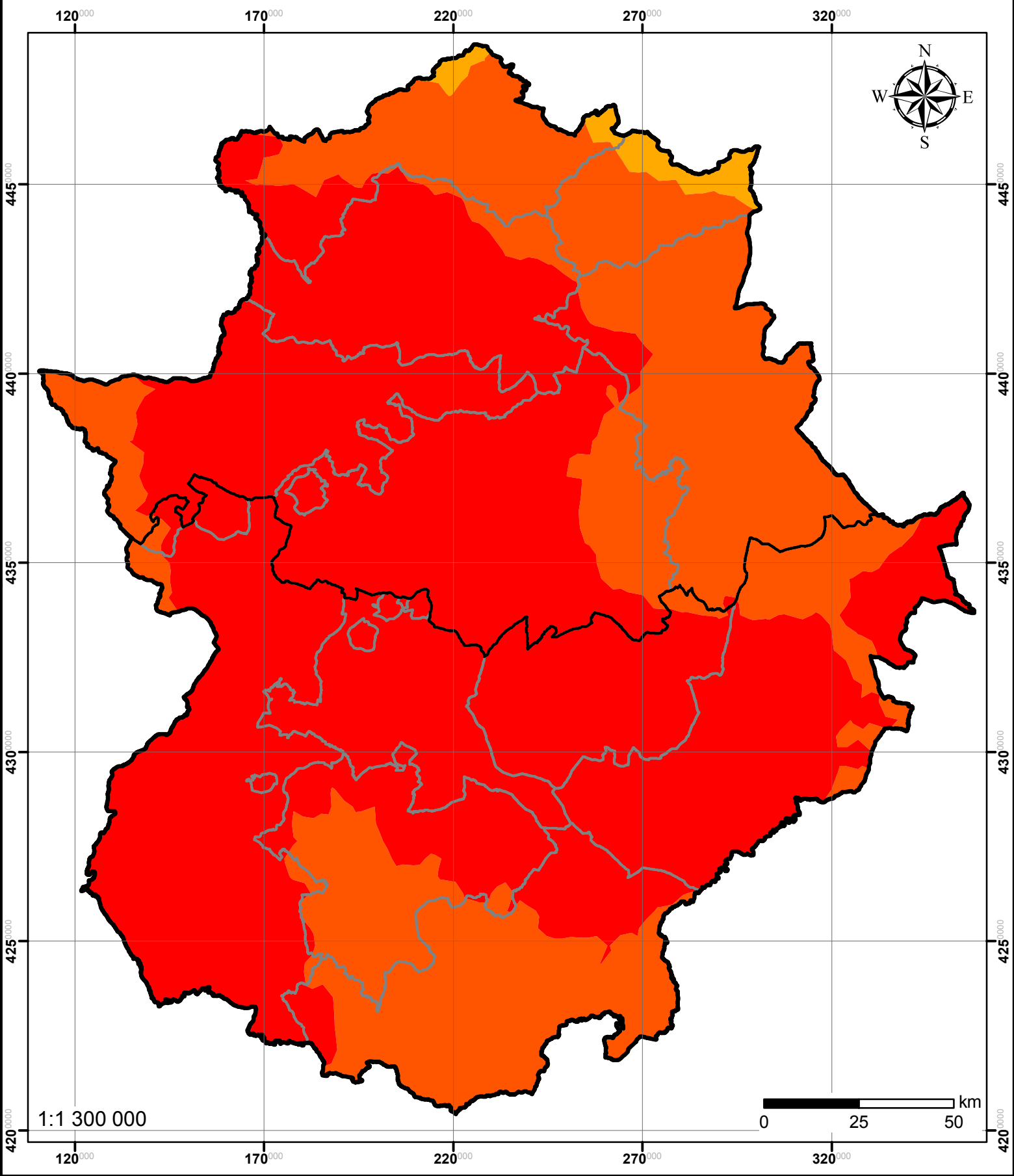
Mapa 5. Temperatura media anual de las máximas diarias del año 2025. Escenario B2.
