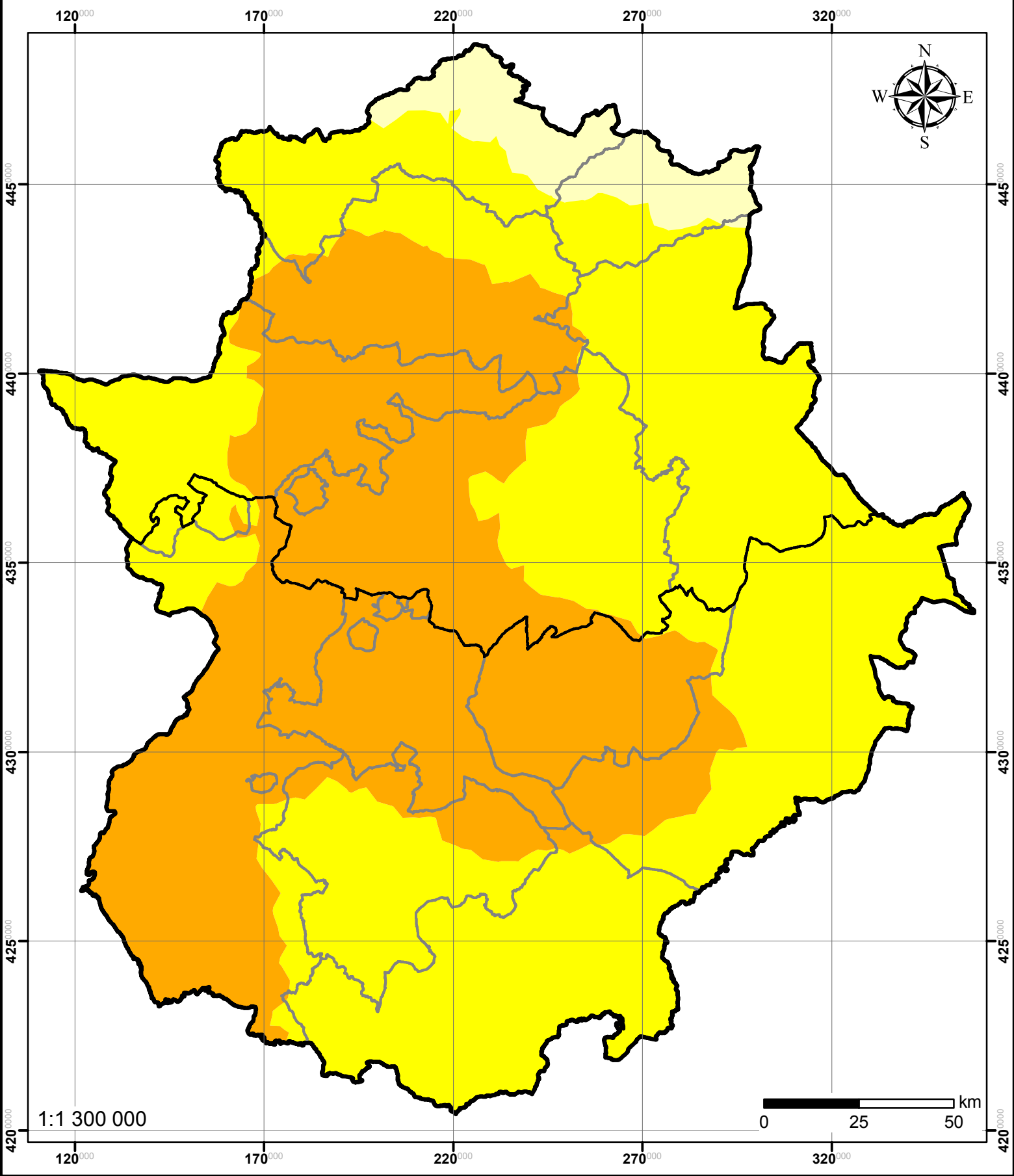
Mapa 3. Temperatura media anual de las máximas diarias del promedio 1961-1990.
