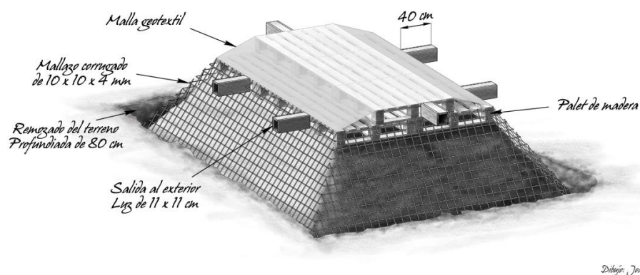
Ilustración 14. Construcción de vivares
