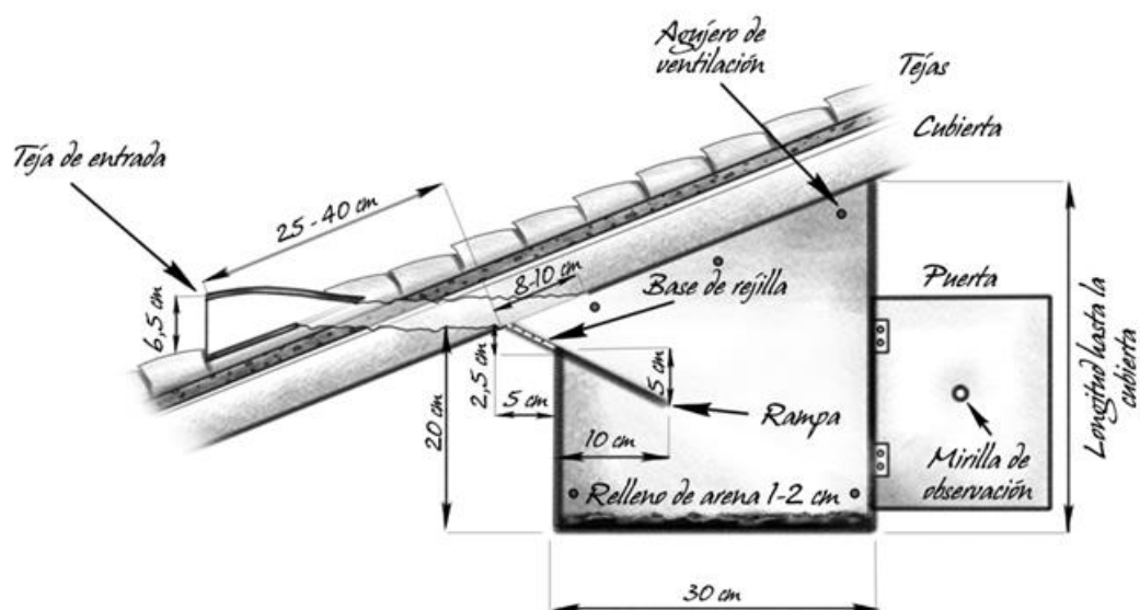
Ilustración 6. Esquema colocación nidal
