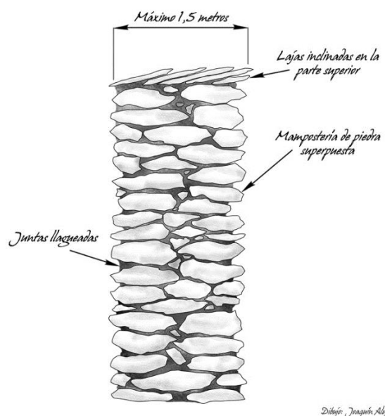
Ilustración 23. Recuperación de elementos históricos del paisaje (muros de piedra)
