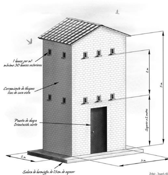
Ilustración 10. Construcción de palomar
