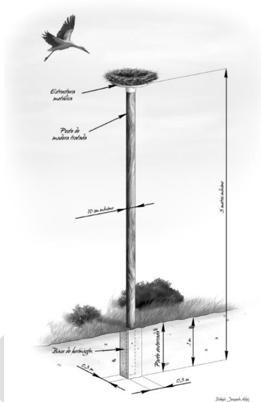
Ilustración 9. Ilustración de un poste de madera con plataforma de nidificación
