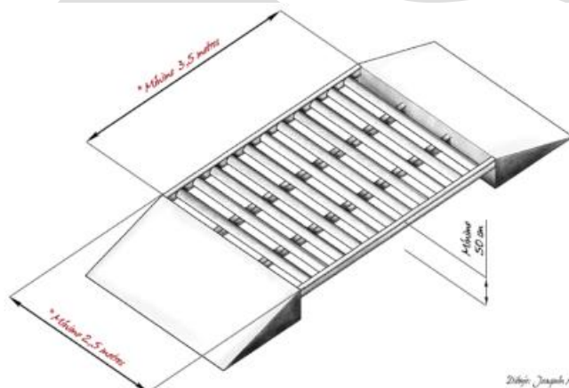
Ilustración 20. Construcción de pasos canadienses no peligrosos para fauna
