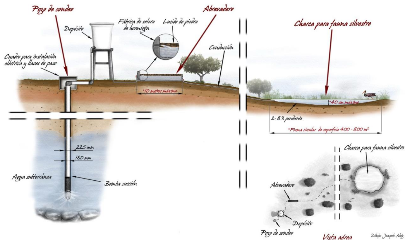
Ilustración 1. Construcción de pozo de sondeo asociado a abrevaderos para evitar uso excesivo de humedales
