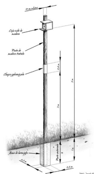
Ilustraciones 11 y 12. Instalación de cajas nido sobre postes
