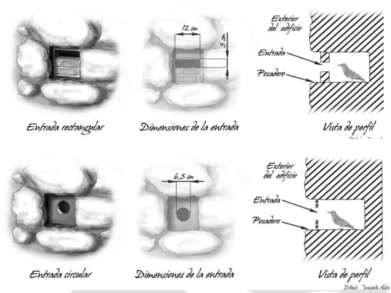
Ilustración 7. Adecuación de huecos en edificios
