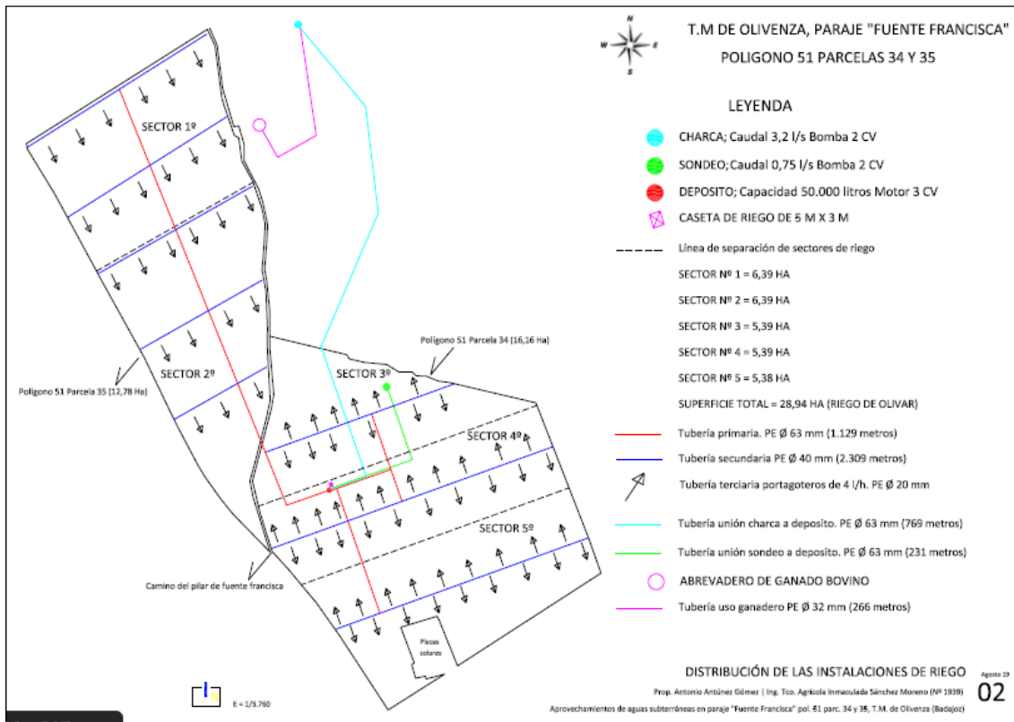
Figura 3. Instalaciones de riego
