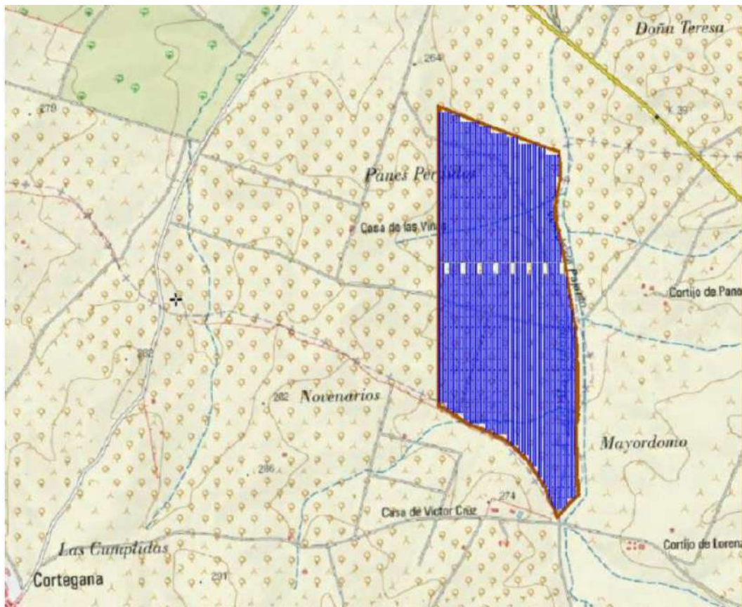
Ilustración 3. Implantación fotovoltaica "Lobón 2"
