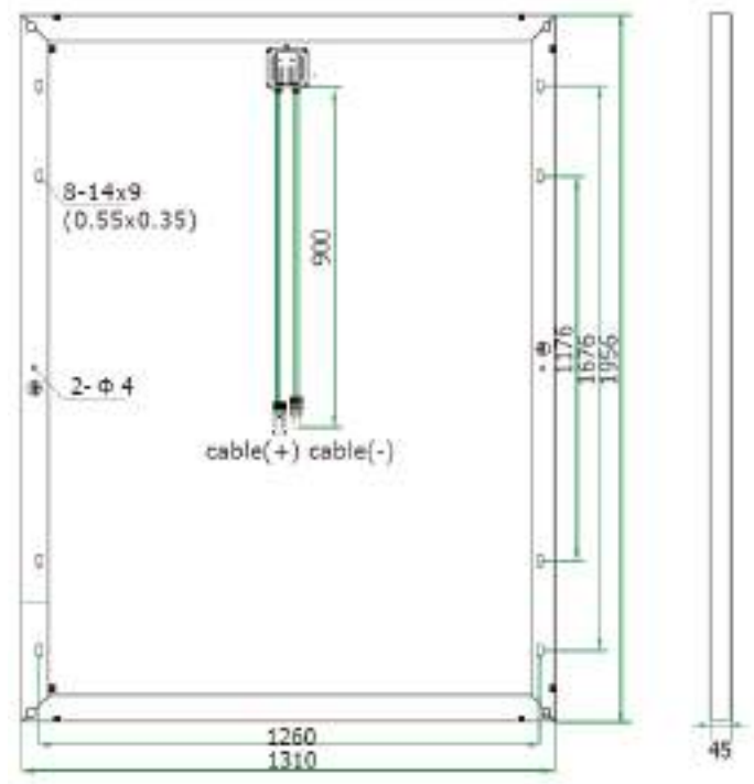
Ilustración 6: Módulo fotovoltaico
