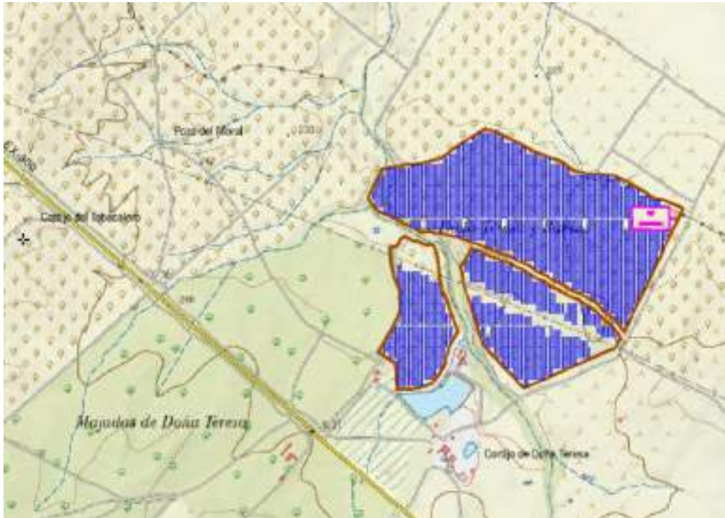
Ilustración 3: Localización planta LOBÓN 1
