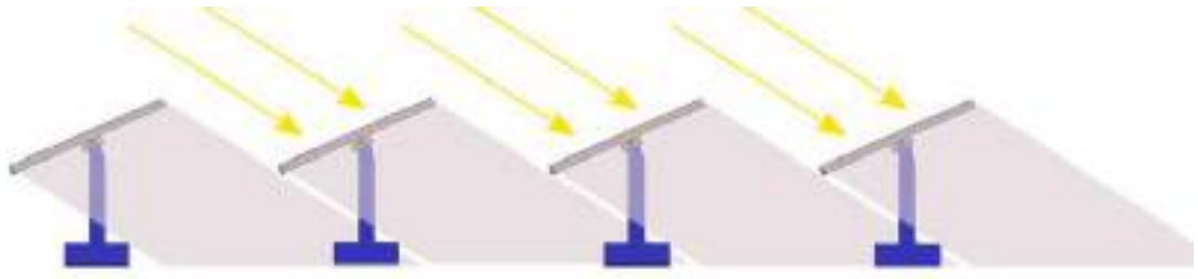
Ilustración 12: Seguidor con backtracking, no se produce sombreado
