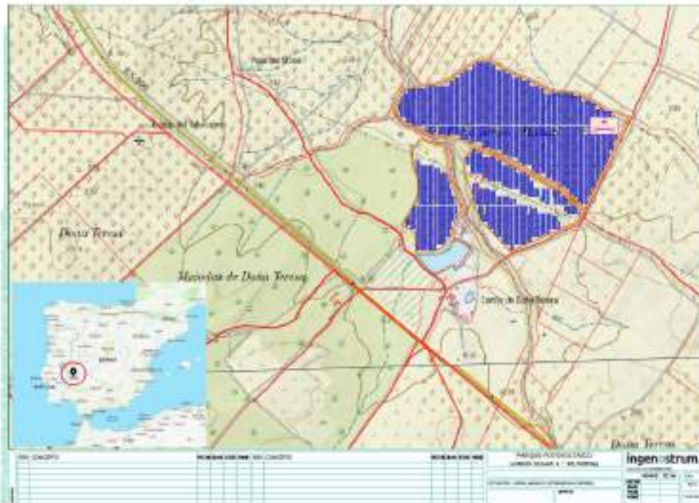
Ilustración 5: Layout general LOBÓN 1
