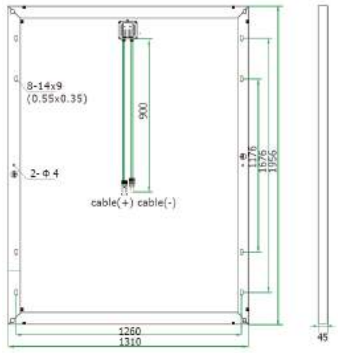
Ilustración 6: Módulo fotovoltaico
