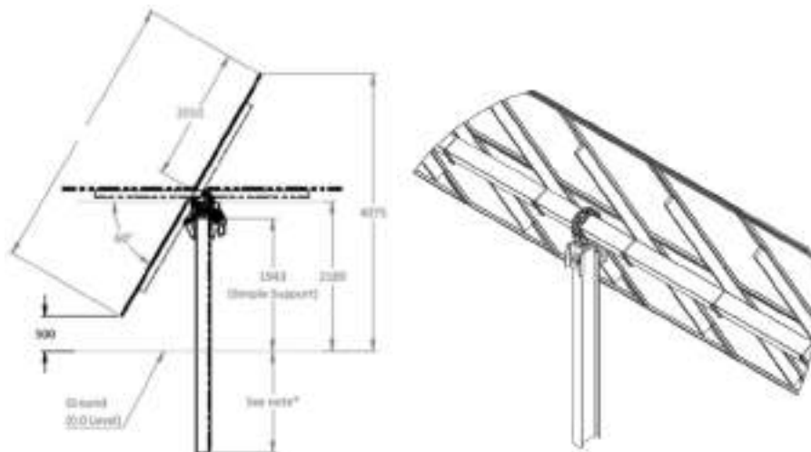
Ilustración 10: Perfil Seguidor Soltec y detalle eje
