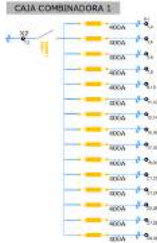
Ilustración 20: Cuadro tipo de agrupación CC inversor de 15 circuitos
