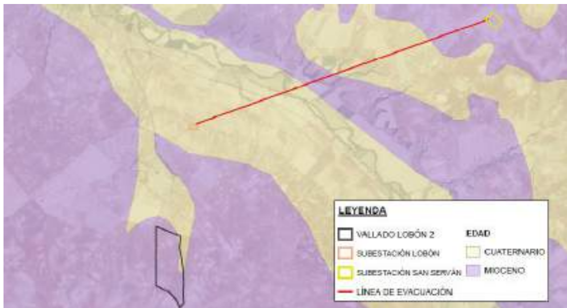
Ilustración 38: Edad del suelo
