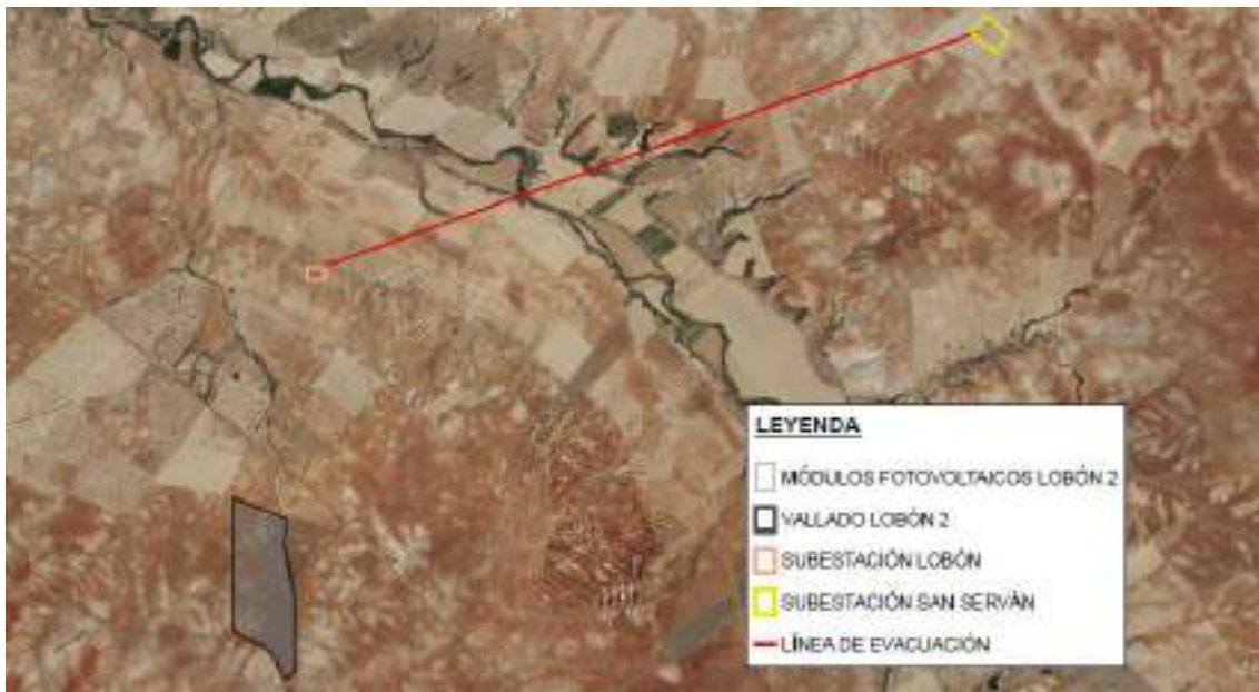
Ilustración 35: Implantación
