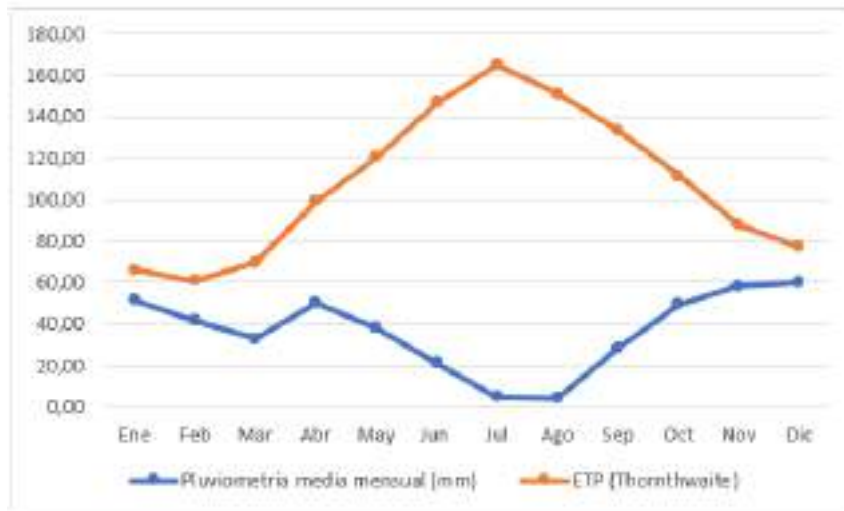
Ilustración 37: Pluviometría y ETP. Elaboración propia
