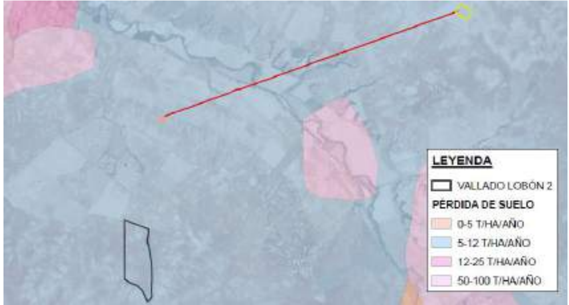
Ilustración 39: Erosión del suelo
